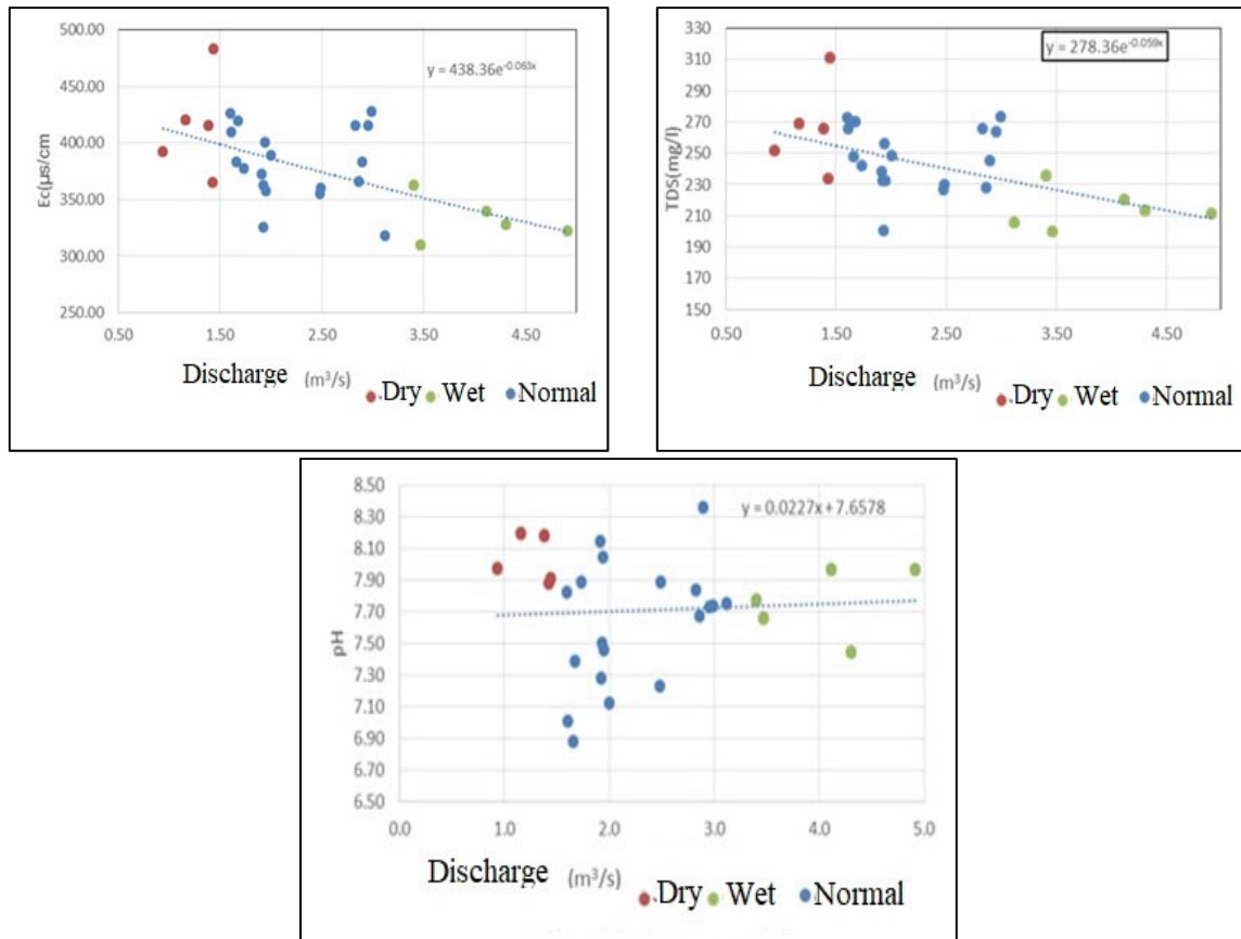
شکل ۵- روابط بین دبی سالانه و پارامترهای کیفیت آب در ایستگاه تنگ محمد حاجی Fig. 5. Relationships between annual discharge and water quality parameters at Tang Mohammad Haji station
