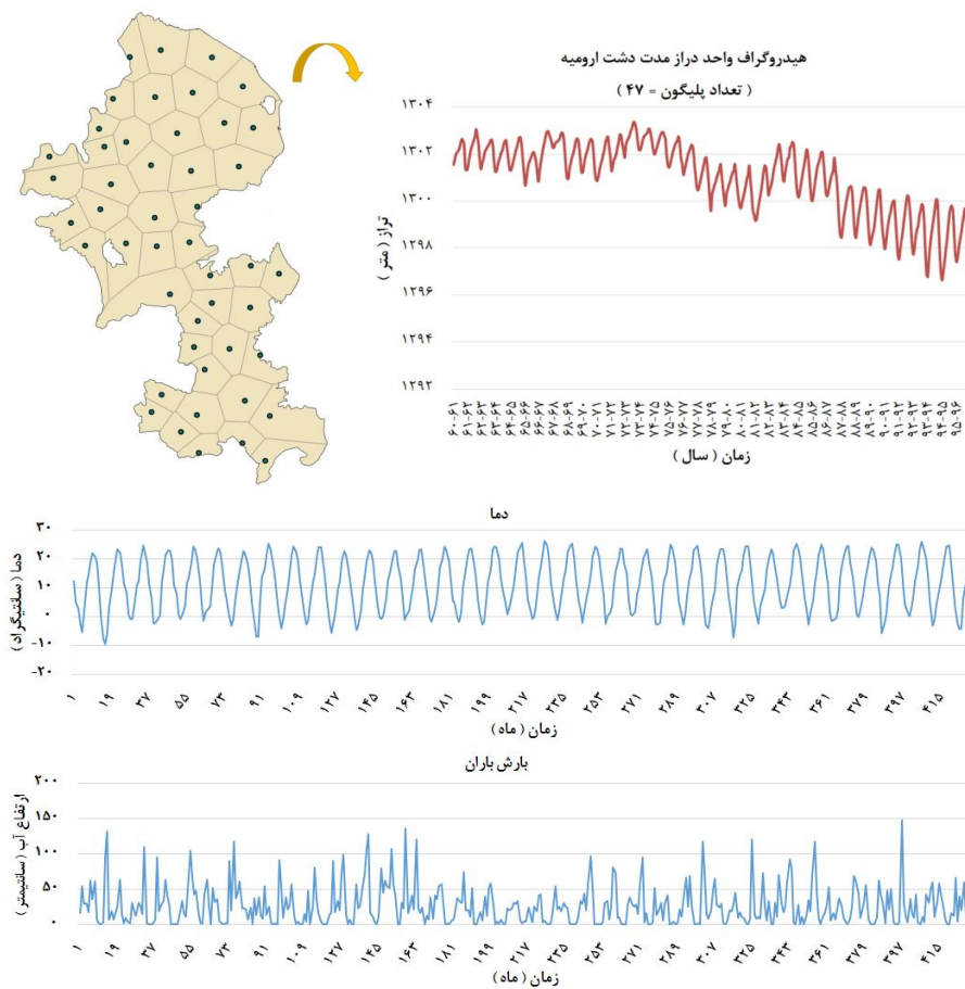
شکل ۴- تیسنبندی و نمودار سطح آب زیرزمینی و دما و بارش متوسط ماهیانه مربوط به ۳۶ سال
