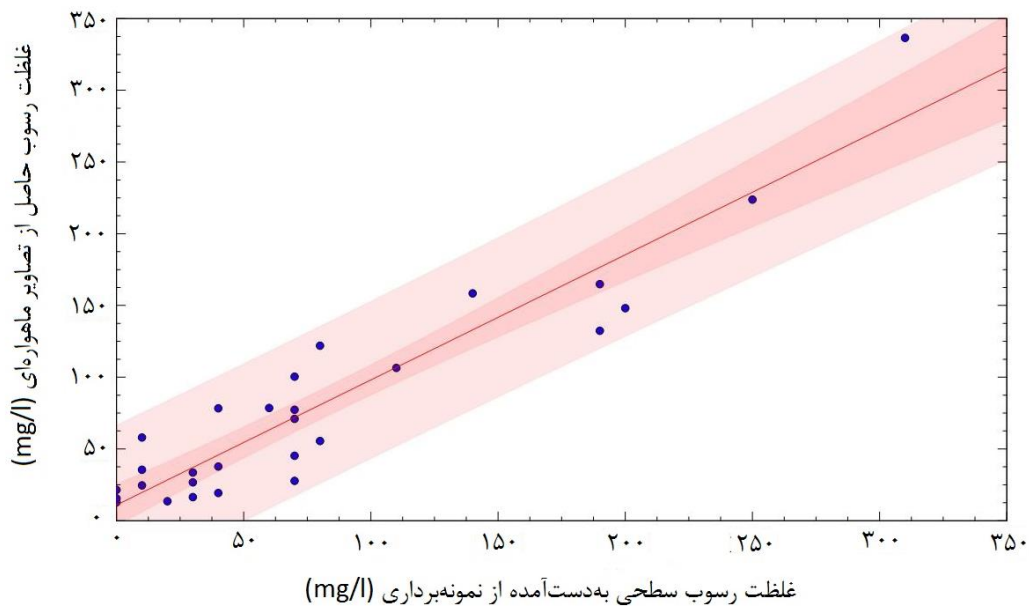
شکل ۶- مقایسه مقدار رسوب به دست آمده از الگوریتم مبتنی بر تصاویر ماهواره‌ای و رسوب سطحی اندازه‌گیری شده
