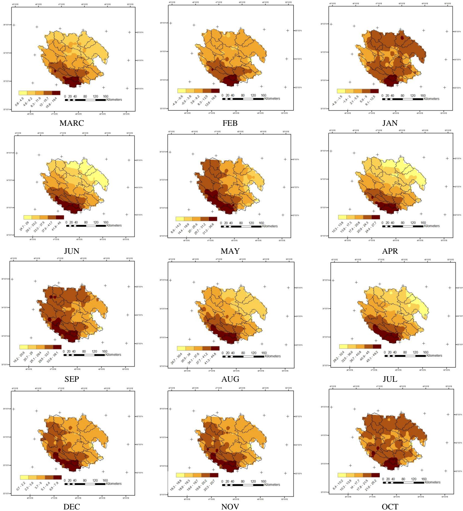
شکل ۵- توزیع مکانی حداکثر ماهانه مشاهده‌ای (درجه سانتی‌گراد)
