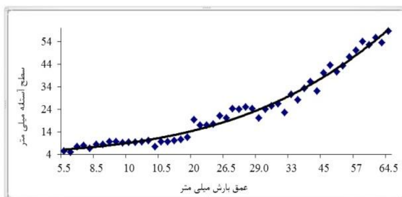
شکل ۹- همبستگی آستانه شروع رواناب با عمق بارش
