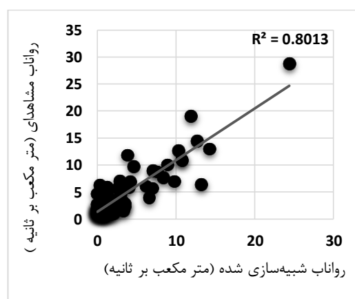
الف- دوره واسنجی رواناب ماهیانه (۲۰۰۲-۲۰۰۸)
