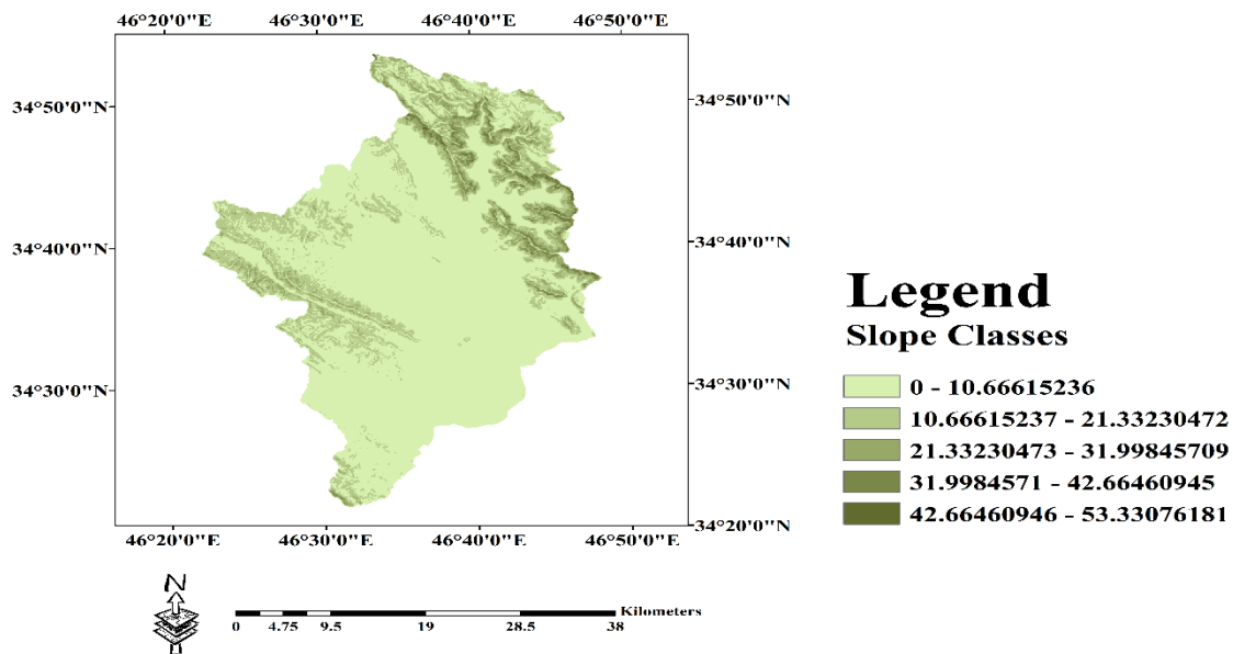
شکل ۳- نقشه شیب حوضه آبخیز روانسر سنجایی
