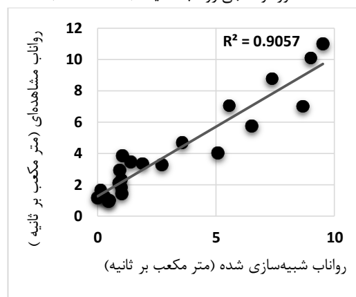
ب- دوره اعتبارسنجی رواناب ماهیانه (۲۰۰۹-۲۰۱۰)
