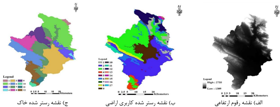
شکل ۴- نقشه‌های رقوم ارتفاعی، کاربری اراضی و خاک حوزه آبخیز روانسر سنجایی
