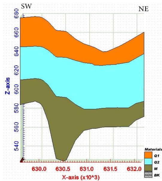
شکل ۱۰- مقطع عرضی در جهت شمال شرق-جنوب غرب ضخامت لایه‌های رسوبات آبرفتی خشک ( Q_2 )، رسوبات آبرفتی احتمالاً آبدار ( Q_1 ) و سنگ کف مارنی (M) به متر
