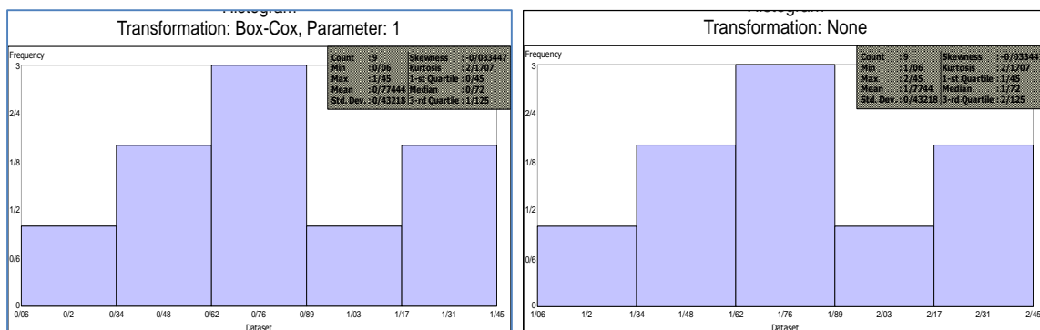
شکل ۴- هیستوگرام ضریب هدایت هیدرولیکی قبل و بعد از نرمال‌سازی
