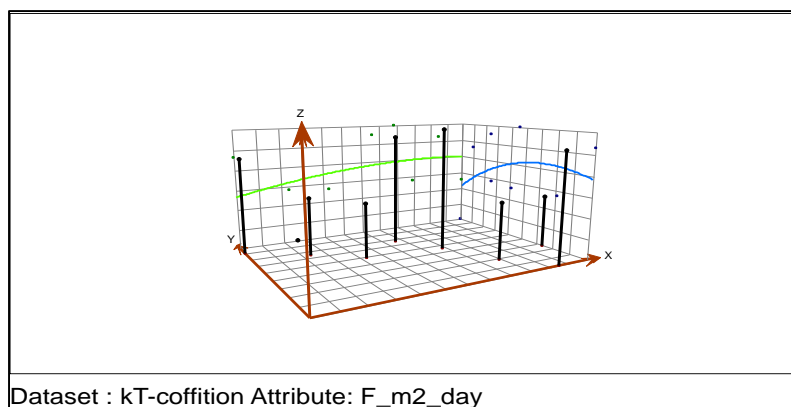
شکل ۸- روند مکانی ضریب قابلیت انتقال نهشته‌های کواترنر
