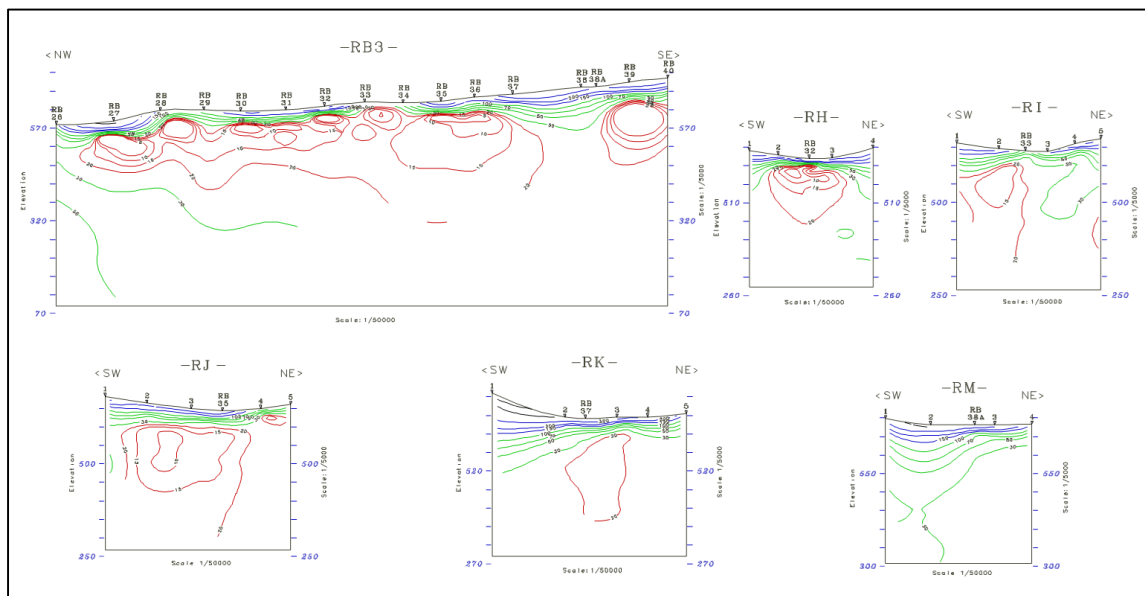
شکل ۱۲- مقاطع هم‌مقاومت ویژه ظاهری دشت جم
