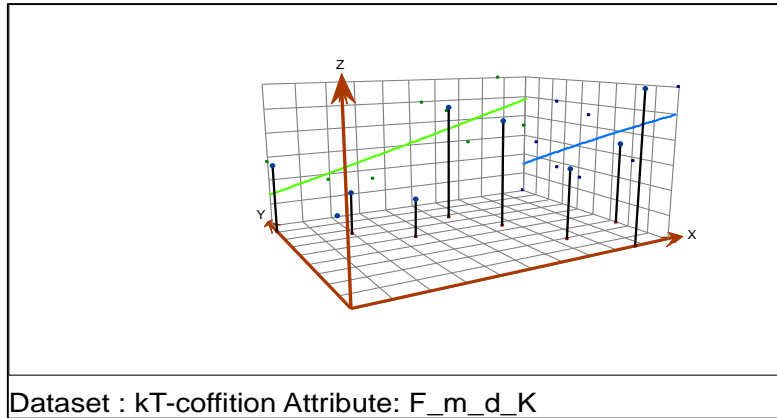
شکل ۵- روند مکانی داده‌های ضریب قابلیت هدایت هیدرولیکی
