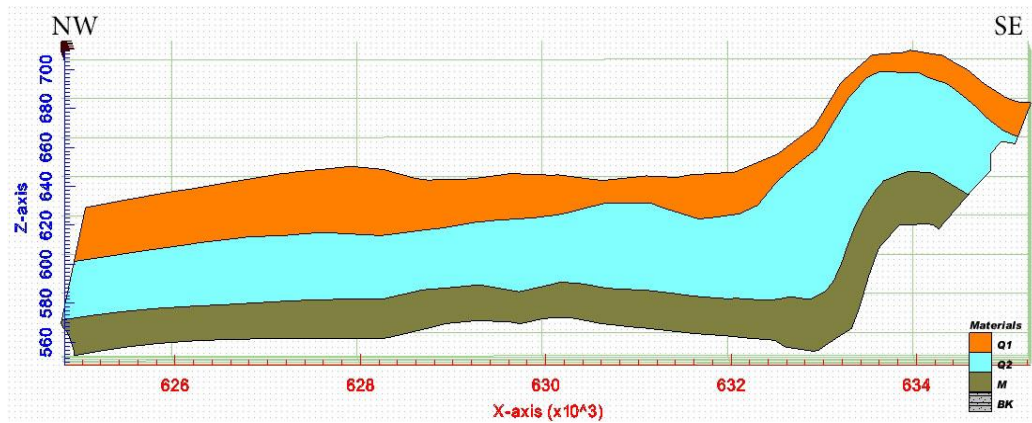
شکل ۱۱- مقطع طولی شمال غربی-جنوب شرقی ضخامت لایه‌های رسوبات آبرفتی خشک (Q 2 )، رسوبات آبرفتی احتمالاً آبدار (Q 1 ) و سنگ کف مارنی (M) به متر
