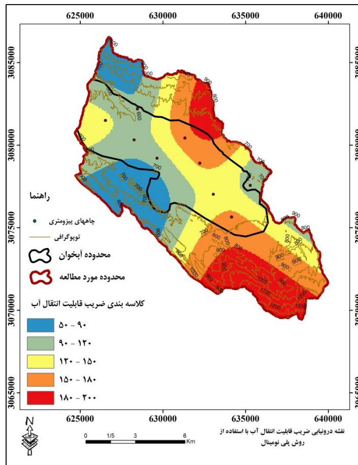
شکل ۹- نقشه درون‌یابی ضریب قابلیت انتقال آب با استفاده از روش پلی‌نومینال
