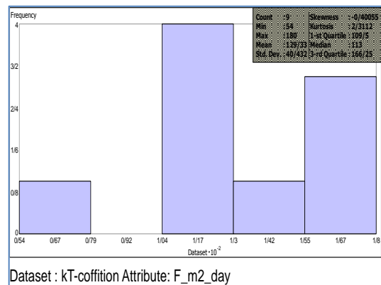
شکل ۷- هیستوگرام داده‌های آماری ضریب قابلیت انتقال قبل و بعد از نرمال‌سازی
