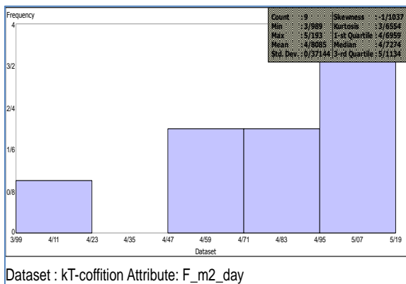
شکل ۷- هیستوگرام داده‌های آماری ضریب قابلیت انتقال قبل و بعد از نرمال‌سازی
