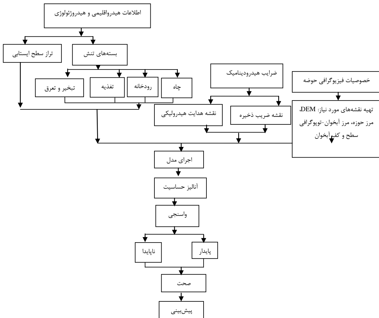
شکل ۲- مراحل اجرای مدل آب زیرزمینی در نرم‌افزار جی ام اس
