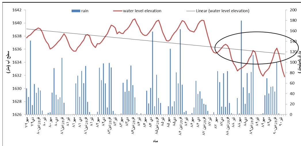
شکل ۴- هیدروگراف معرف دشت تویسرکان (سال‌های واسنجی و اعتبارسنجی با دایره نشان داده شده است)
